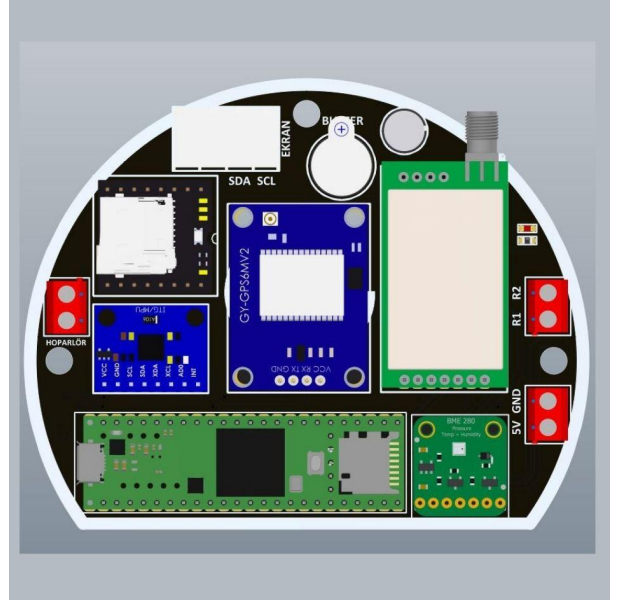
3.1 Uçu bilgisayar ana kartı
